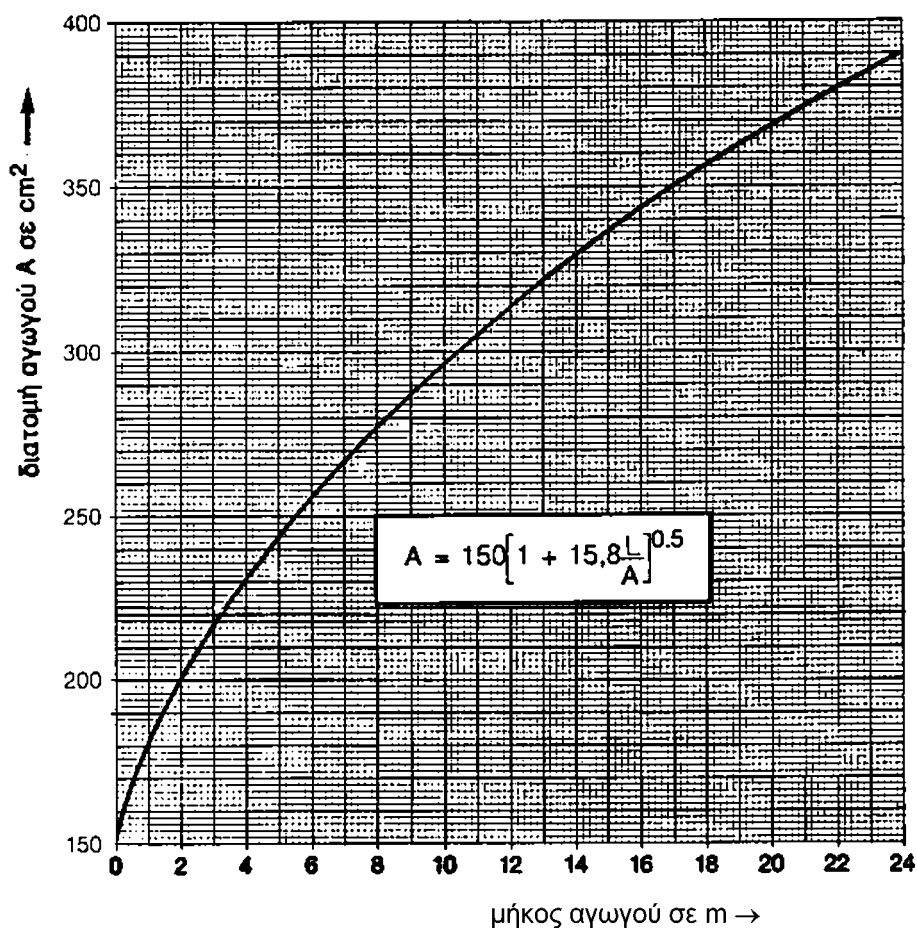
Διάγραμμα 10.1 Ισοδύναμη τετράγωνη διατομή αγωγού για αγωγό ελεύθερης διατομής 150 \text{ cm}^2 εξαρτώμενη από το μήκος του αγωγού L
